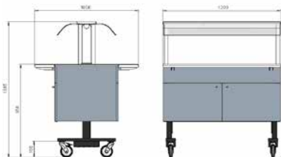
120 - höjd 950 mm Ø125 mm
